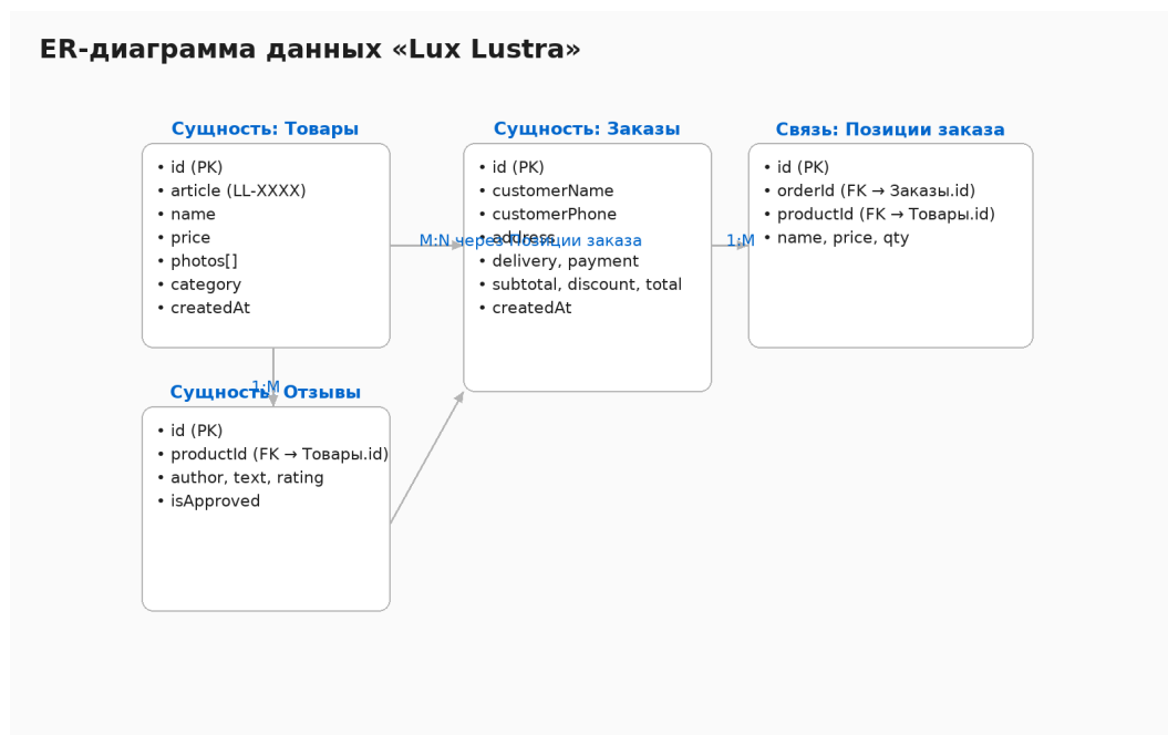
Рисунок 2 – ER-диаграмма базы данных
