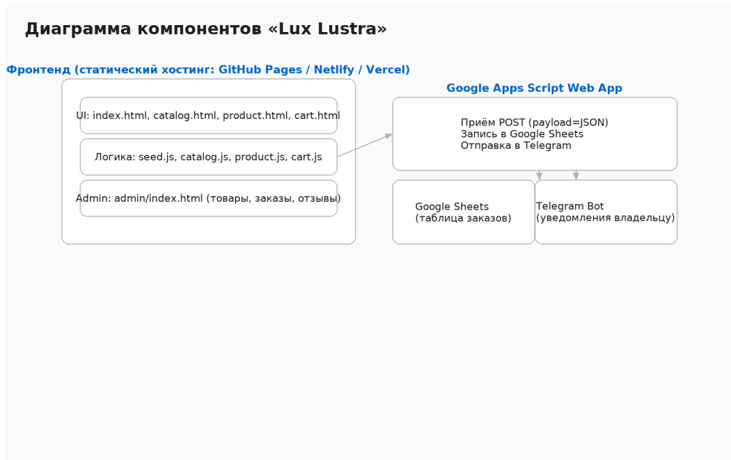
Рисунок 3 – Диаграмма компонентов
